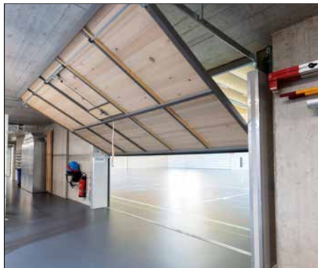
Geräteraumtor mit zwei-Punkt-Verriegelung und gefederten Schliessriegeln.
